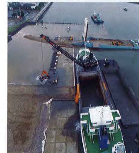
施工状況
