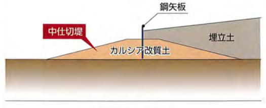
中仕切堤部 断面図
