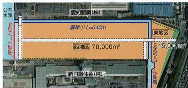
■ 施工位置図
