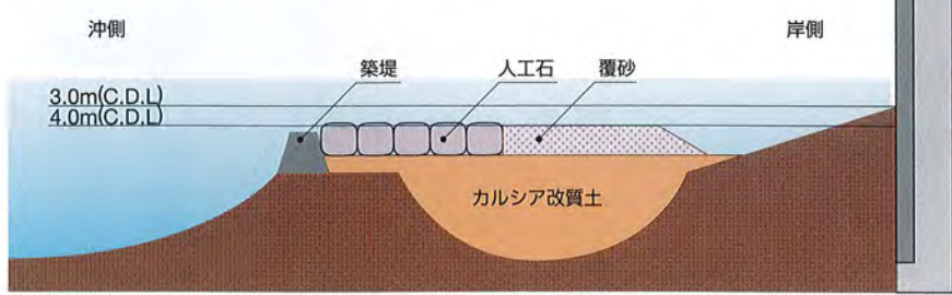
■ 浅場の断面図 (平成23年施工区を例に)
