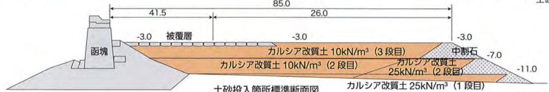
土砂改良工
